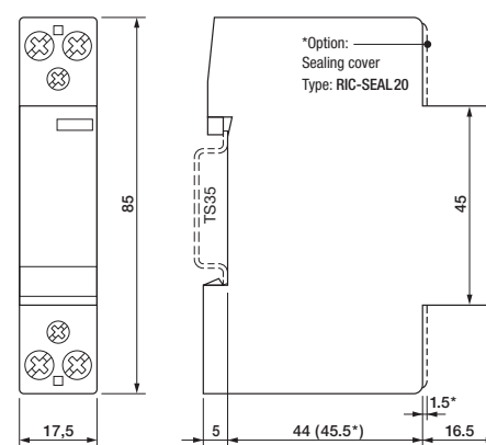
fig. 3. Abmessungen (mm)
