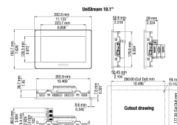
fig. 1. Abmessungen (mm)
