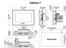
fig. 1. Abmessungen (mm)
