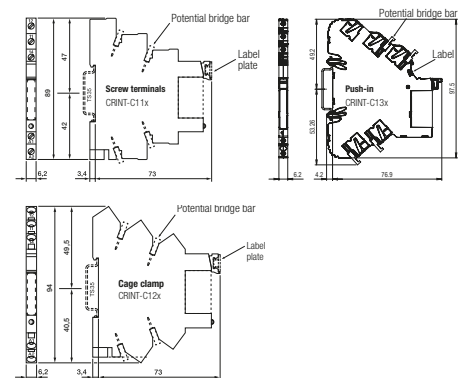
fig. 3. Dimensions (mm)
