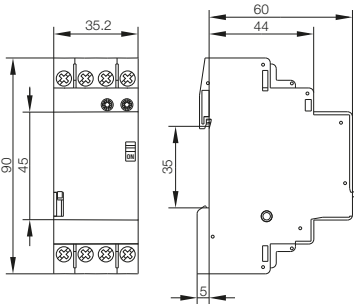
fig. 3. Dimensions (mm)
