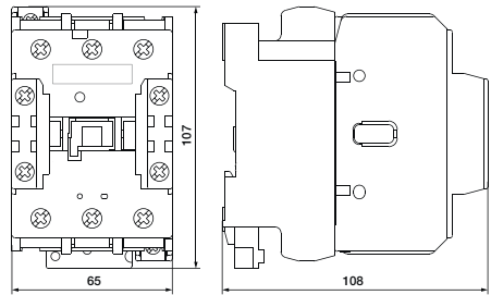
fig. 3. Dimensions (mm)
