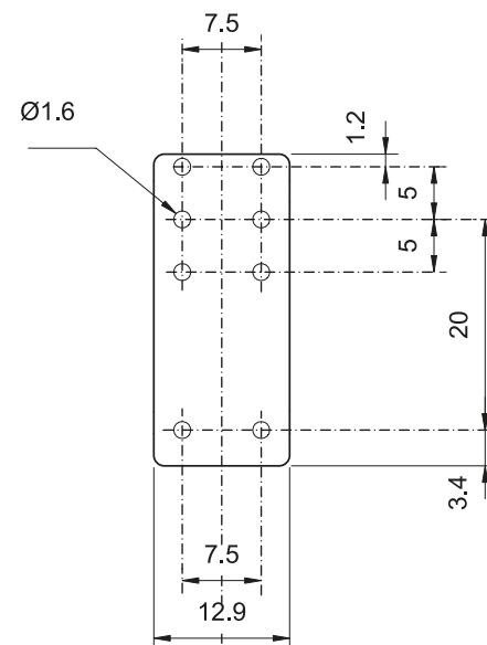
fig. 2. Abmessungen (mm)
