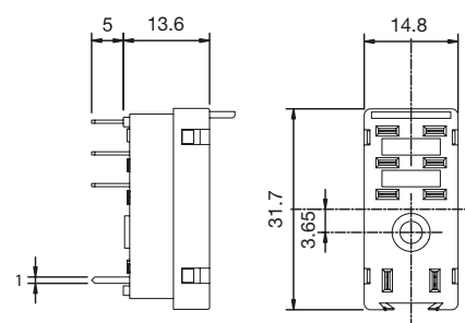
fig. 2. Abmessungen (mm)
