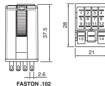
fig. 4. Dimensions (mm)
