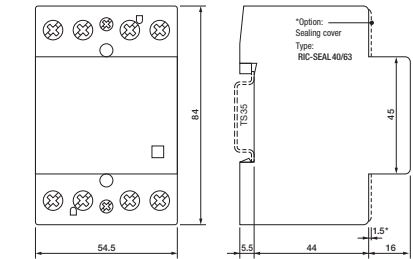
fig. 3. Dimensions (mm)
