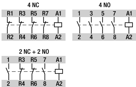
fig. 1. Wiring diagram
