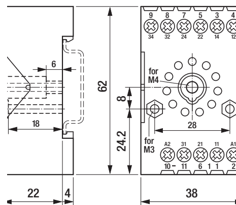
fig. 2. Abmessungen (mm)
