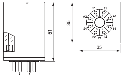
fig. 4. Dimensions (mm)
