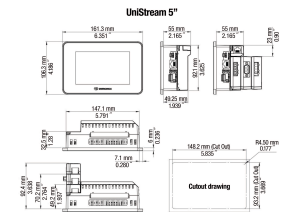
fig. 1. Dimensions (mm)
