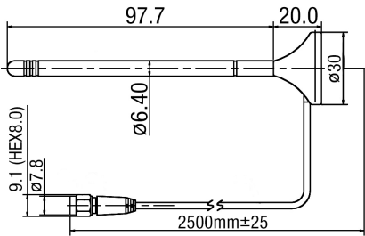
fig. 1. Abmessungen (mm)
