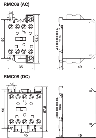
fig. 3. Dimensions (mm)
