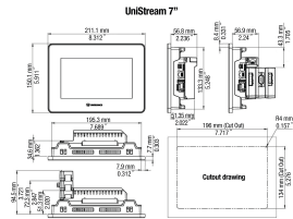
fig. 1. Dimensions (mm)
