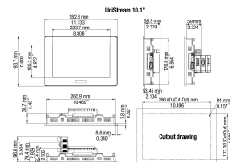
fig. 1. Dimensions (mm)
