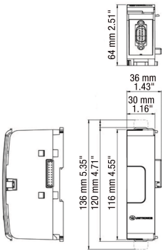
fig. 1. Dimensions (mm)
