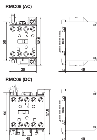
fig. 3. Abmessungen (mm)
