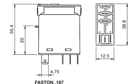
fig. 4. Dimensions (mm)
