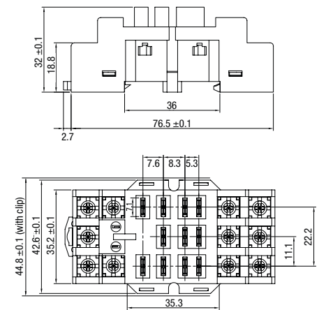
fig. 2. Abmessungen (mm)
