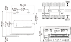
fig. 1. Dimensions (mm)
