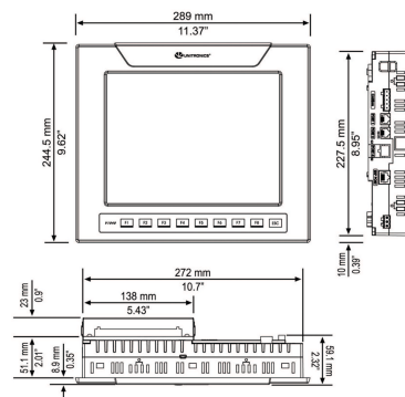
fig. 1. Abmessungen (mm)
