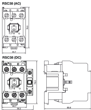
fig. 3. Dimensions (mm)
