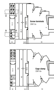
fig. 4. Dimensions (mm)
