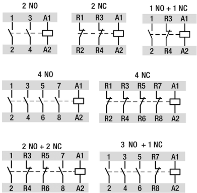
fig. 1. Wiring diagram
