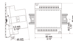
fig. 1. Dimensions (mm)
