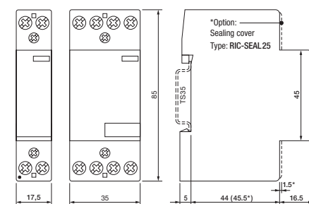
fig. 3. Abmessungen (mm)
