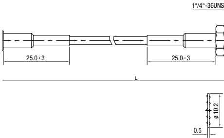
fig. 2. Abmessungen (mm)
