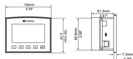
fig. 1. Dimensions (mm)
