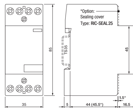
fig. 3. Dimensions (mm)
