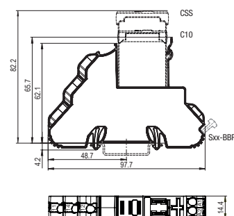
fig. 4. Dimensions (mm)
