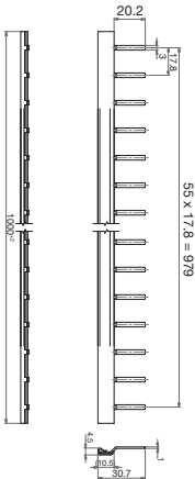
fig. 1. Abmessungen (mm)
