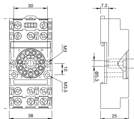
fig. 2. Abmessungen (mm)
