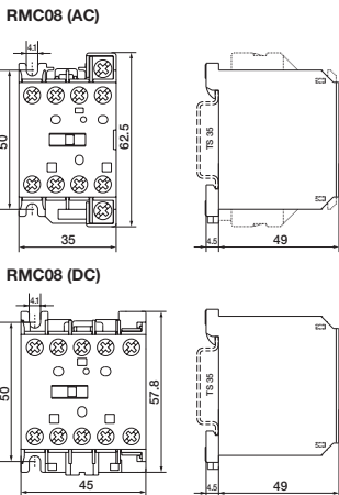
fig. 3. Dimensions (mm)
