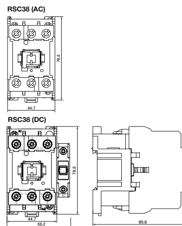
fig. 3. Abmessungen (mm)
