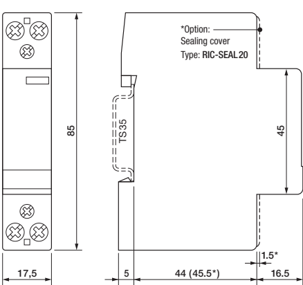
fig. 3. Dimensions (mm)
