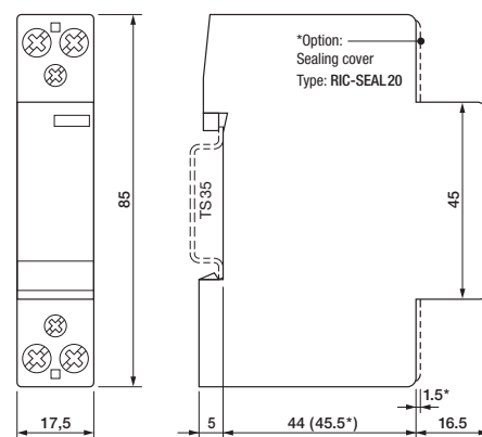
fig. 3. Dimensions (mm)
