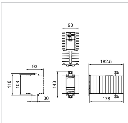
«Massbild d» 90 mm Modul
