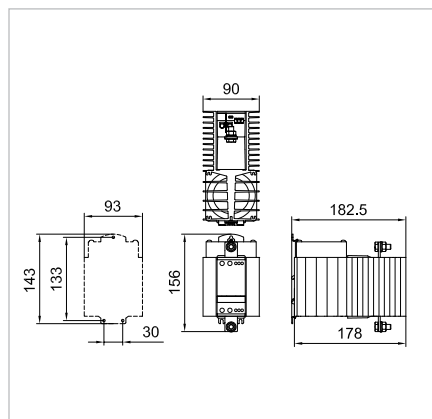
«Massbild e» 90 mm Modul mit Lüfter
