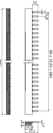
fig. 1. Abmessungen (mm)
