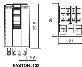
fig. 4. Dimensions (mm)
