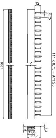
fig. 1. Dimensions (mm)
