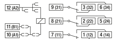
fig. 1. Wiring diagram
