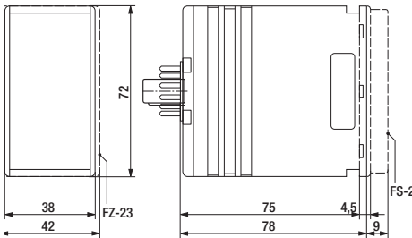
fig. 4. Dimensions (mm)
