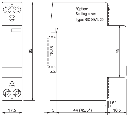
fig. 3. Dimensions (mm)
