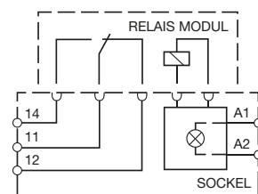
fig. 2. Wechselstrom-Schaltzyklen
