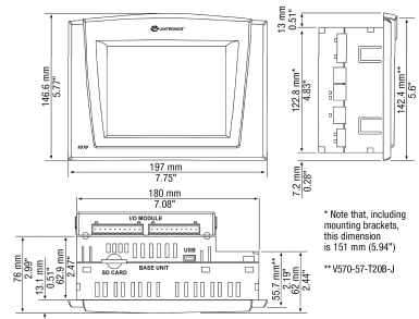
fig. 1. Dimensions (mm)
