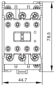
fig. 3. Abmessungen (mm)
