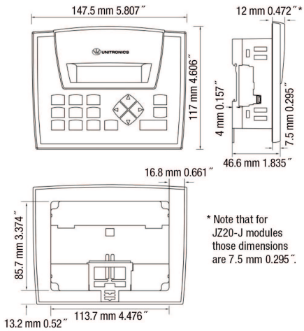
fig. 1. Dimensions (mm)
