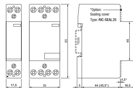
fig. 3. Dimensions (mm)
