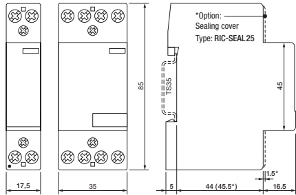
fig. 3. Dimensions (mm)
