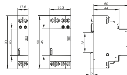
fig. 3. Dimensions (mm)
