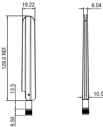
fig. 1. Dimensions (mm)
